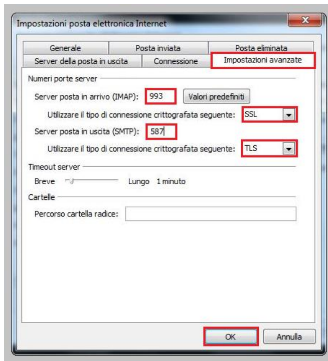
Figura 17 – Configurazione porte
