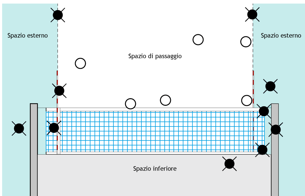
Figura 5a - Spazio di passaggio - R. 2.4, 8.4.3, 8.4.4, 8.4.5, 10.1.1, 10.1.3, 23.3.2.3f, 24.3.2.1, 24.3.2.7, 29.2.1.3, 29.2.1.7
