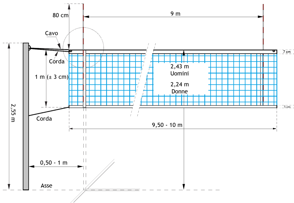
Figura 3a - Disegno della rete - R. 2.1.1, 2.2, 2.3, 2.4, 2.5.1, 8.4.3, 11.3.1, 11.3.2, 29.2.1.6
